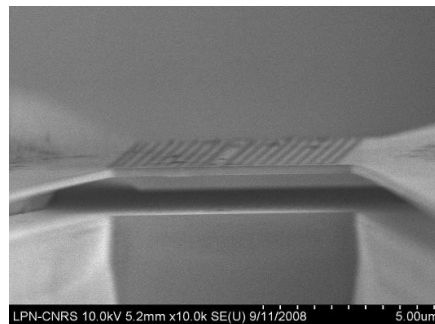
Cliché au microscope électronique à balayage de la membrane suspendue employée comme oscillateur optique et mécanique.
