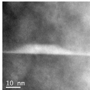
Cliché au microscope électronique en transmission d'une boîte quantique unique d'InAsP sur InP
