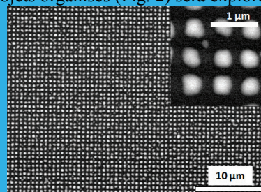
Figure 2: Réseau de nanoparticules d'Ag obtenues par démoillage à l'état solide sur des surfaces de silice structurées par nano-impression.
