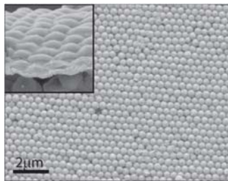
Cristal plasmonique
