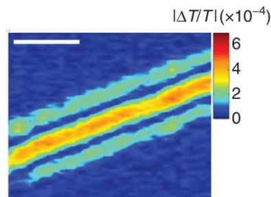
Détection optique d'un nanotube de carbone individuel (ref. 2)
