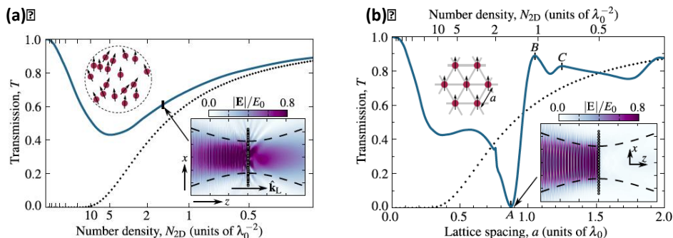
Figure - Prédiction théorique de la transmission de la lumière par un plan d'atomes froids désordonnés (a) et ordonné selon une structure triangulaire (b). Pour une distance entre les atomes de l'ordre de 0.9\lambda , la transmission est parfaite et la réflexion nulle. Figures tirées de [Bettles (PRL 2016)].
